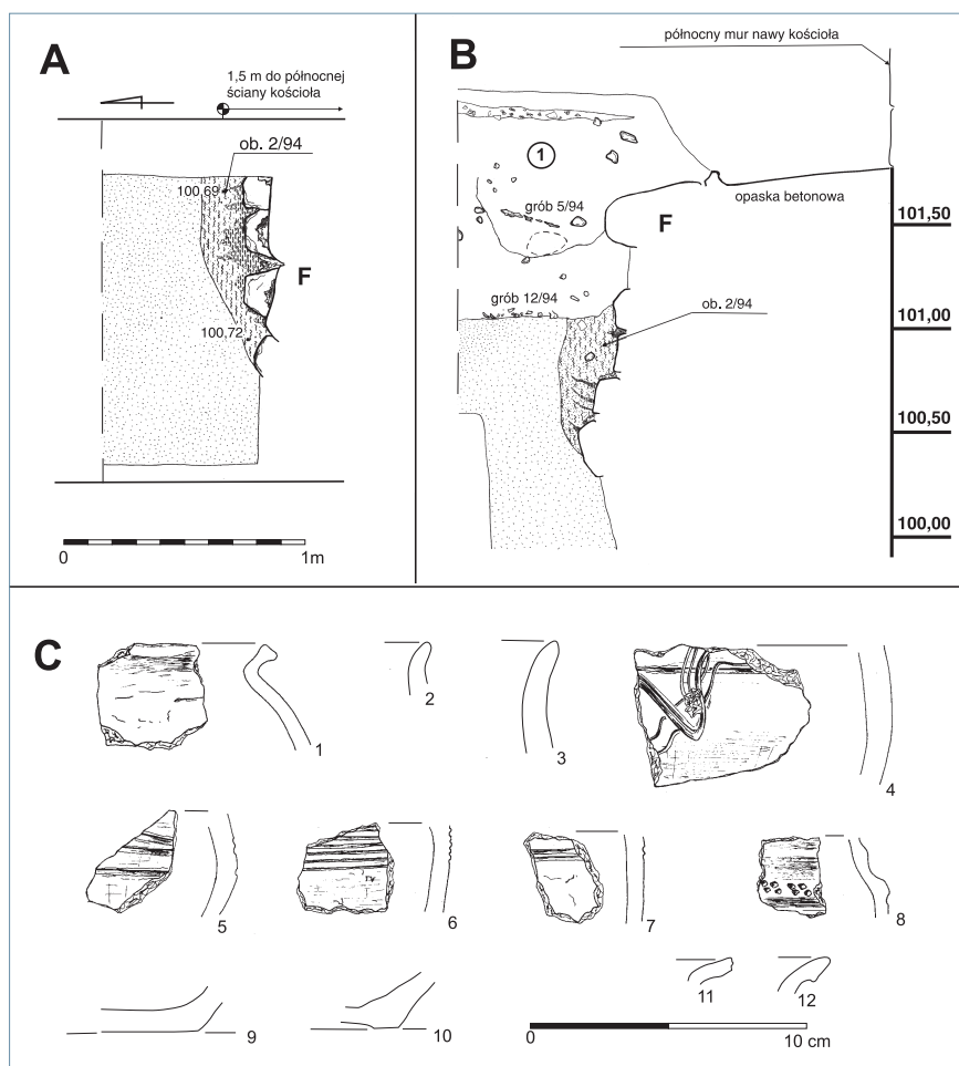
RYCINA 9 Giecz, stan. 3. Obiekt 2/94 (A — rzut poziomy obiektu; B — przekrój obiektu w ścianie wschodniej wykopu; C — ceramika naczyniowa z obiektu; F — fundament północnego muru nawy kościoła I fazy); legenda — por. ryc. 8 (rys. T. Kryštofiak)
