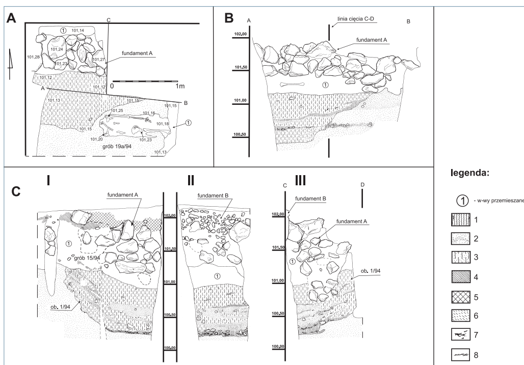
RYCINA 7 Giecz, stan. 3; obiekt 1/94. A — zarys stropu, B — przekrój obiektu wzdłuż linii A-B; C — przekroje obiektu (I — w ścianie zachodniej wykopu, II — w ścianie północnej wykopu; III — wzdłuż linii cięcia C-D). Legenda: 1 — próchnica; 2 — piasek; 3 — piasek z domieszką próchnicy; 4 — glina; 5 — polepa przemieszana z próchnicą; 6 — margiel; 7 — spalenizna; 8 — popiół (rys. T. Krysztofiak)
