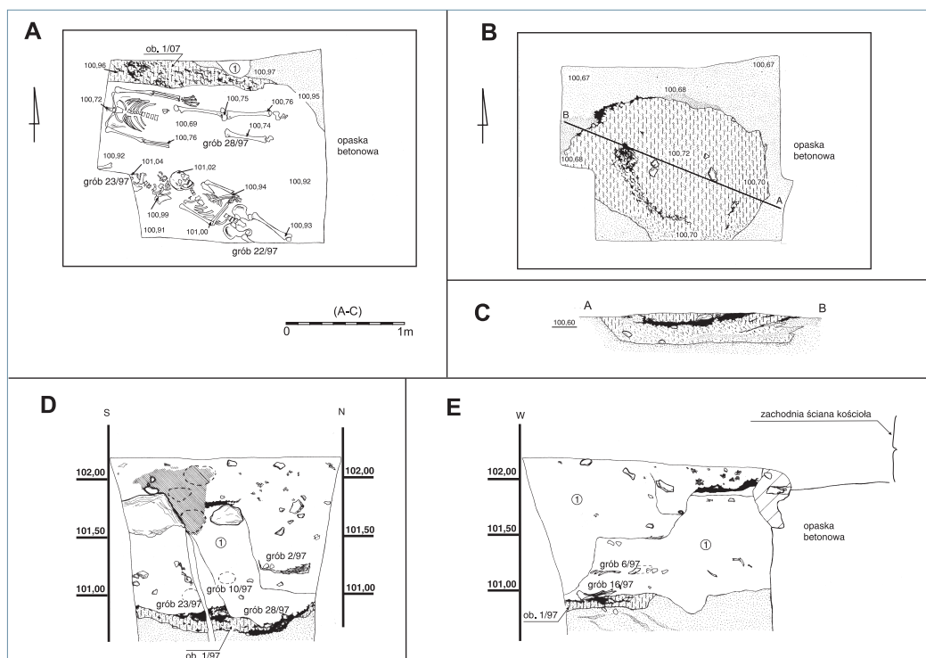
RYCINA 11 Giecz, stan. 3; obiekt 1/97. A — strop obiektu zniszczony wkopami grobowymi; B — zarys obiektu po zdjęciu grobów; C — przekrój obiektu wzdłuż linii A–B; D — przekrój obiektu w ścianie zachodniej wykopu; E — przekrój obiektu w ścianie północnej wykopu; legenda — por. ryc. 8 (rys. T. Krysztofiak)
